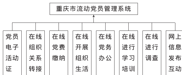
图 1 重庆流动党员管理系统功能图
