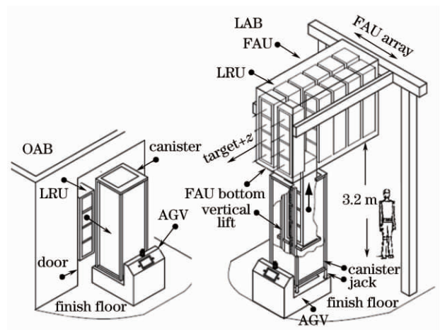
图3 设备设计方案与实现示意。
