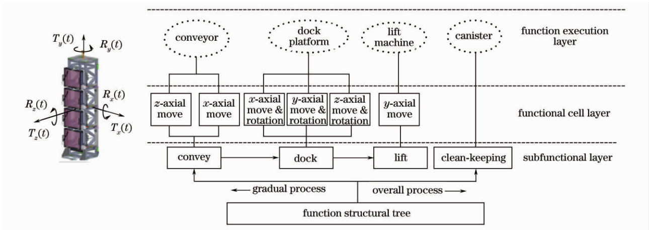
图 2 现场安装工艺设备功能结构树
