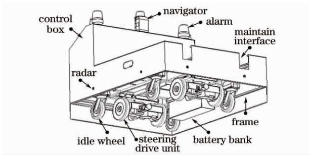
图4 AGV结构设计布局
