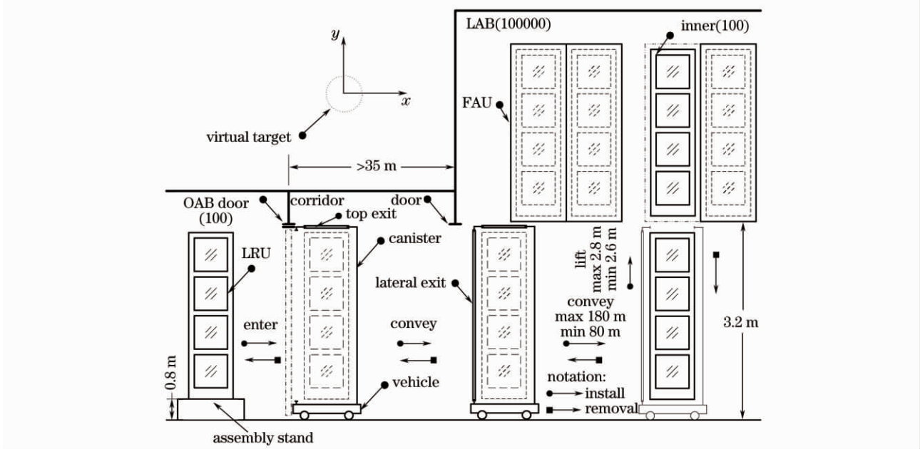
图 1 LRU 现场安装的空间布局与安装示意
